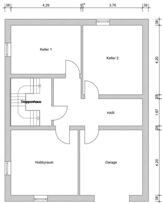
Kellergeschoss
