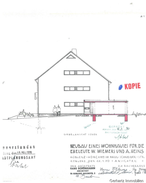
Ansicht-Giebel-Süden
