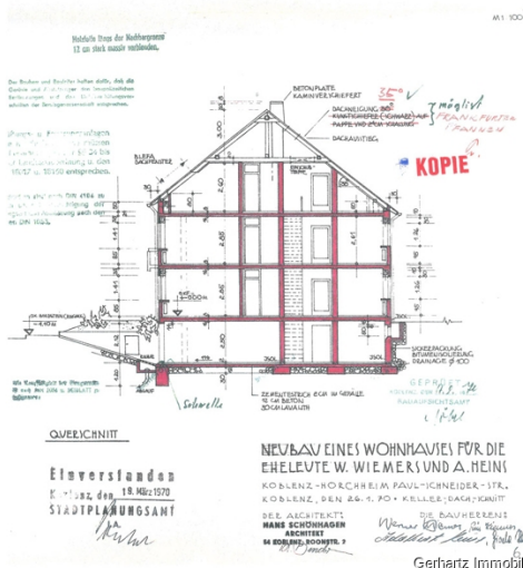
Querschnitt
